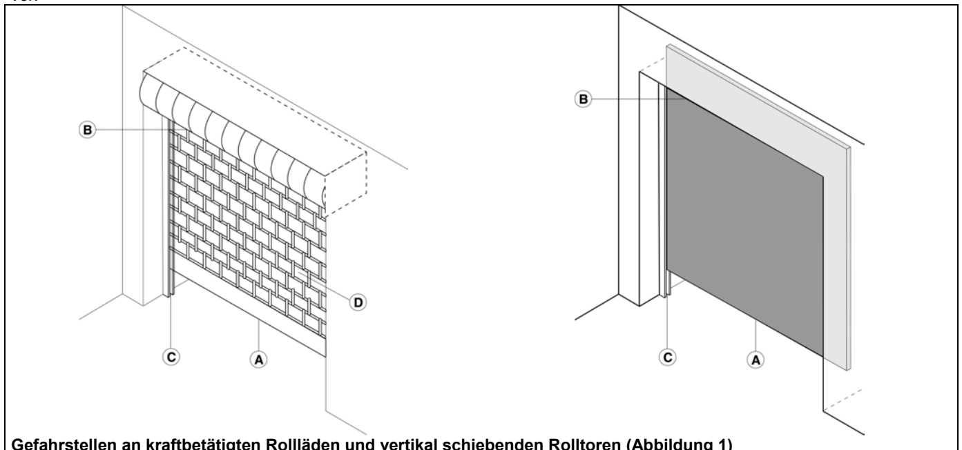
Gefahrstellen an kraftbetätigten Rollläden und vertikal schiebenden Rolltoren (Abbildung 1)
